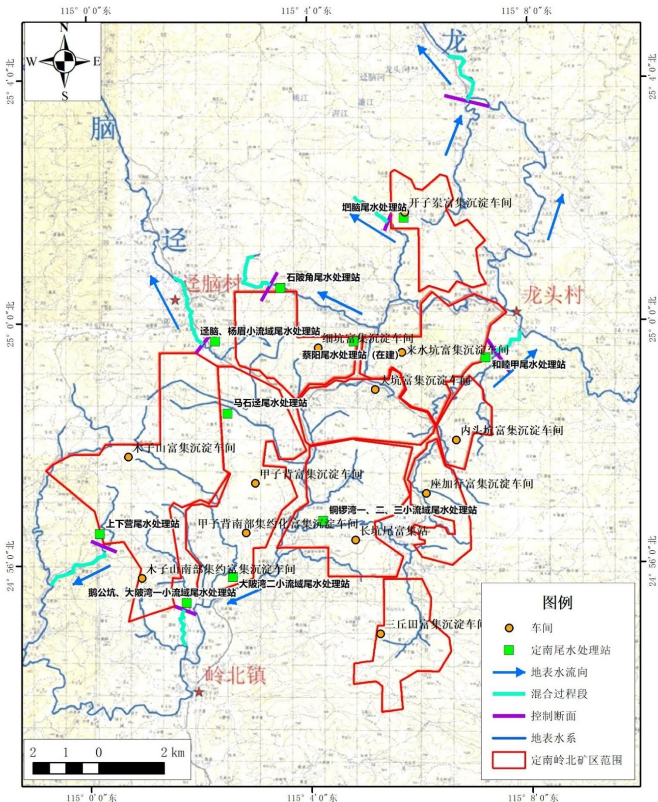
图 6.4-1 定南岭北矿区地表水系及评价标准体系图
