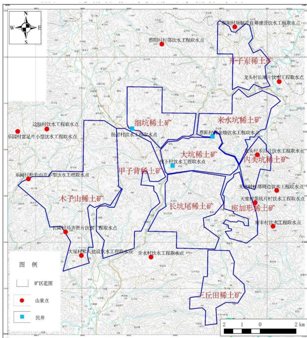
图 6.5-1 定南岭北矿区地下水保护目标图
