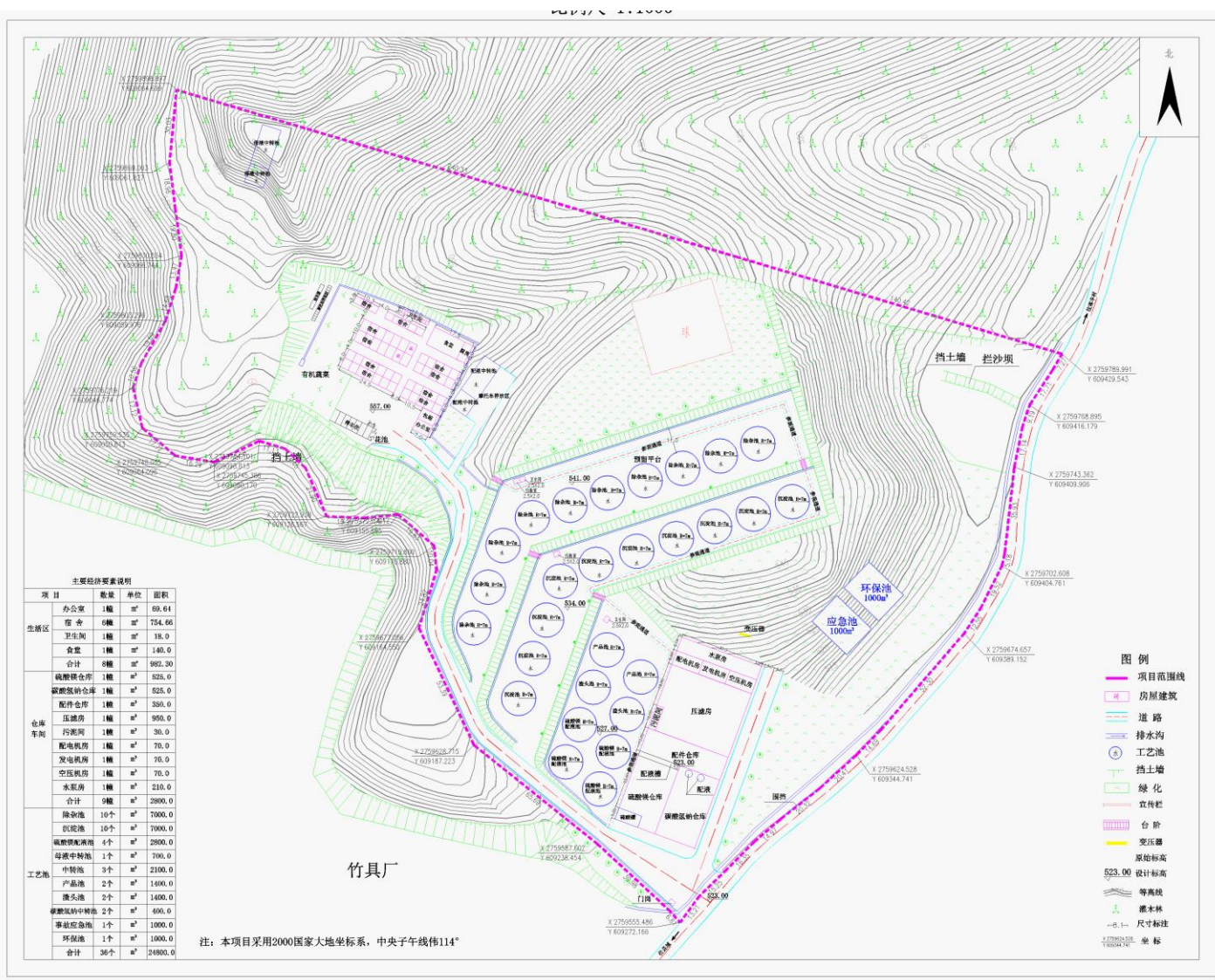
图 3.3-2 长坑尾富集沉淀车间平面布置图
